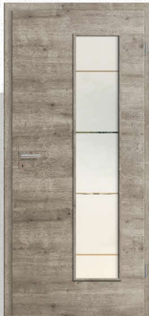
CPL Puristo Alaska Eiche astig quer Lichtausschnitt LV bandseitig Glas Siero 02 Siebdruck Rosettengarnitur Viona Quadro OF 60 Zarge Sinus 60
